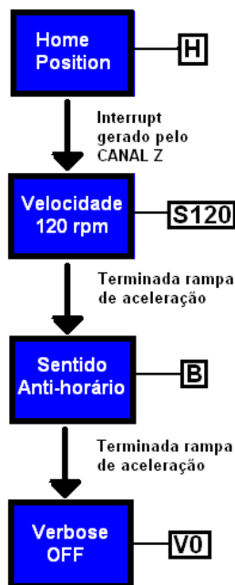
Figura 61: Diagrama para exemplo de instrução
