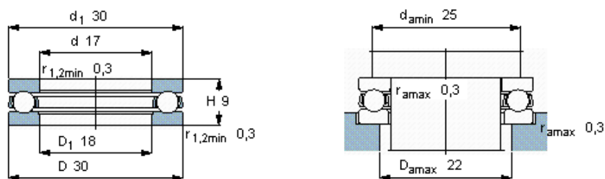
Figura 29: Dimensões do rolamento axial de esferas 51103
